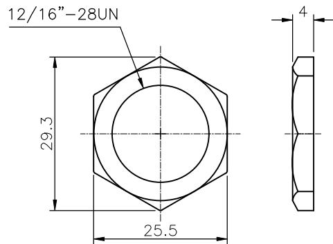
Hex Nut
