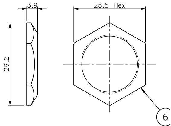
Nut
