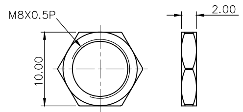
NUT
